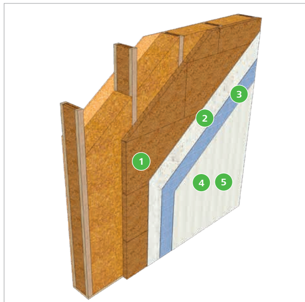
Ossature bois avec contreventement intérieur
