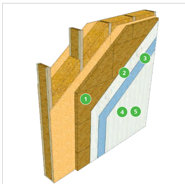
Ossature bois avec contreventement extérieur
